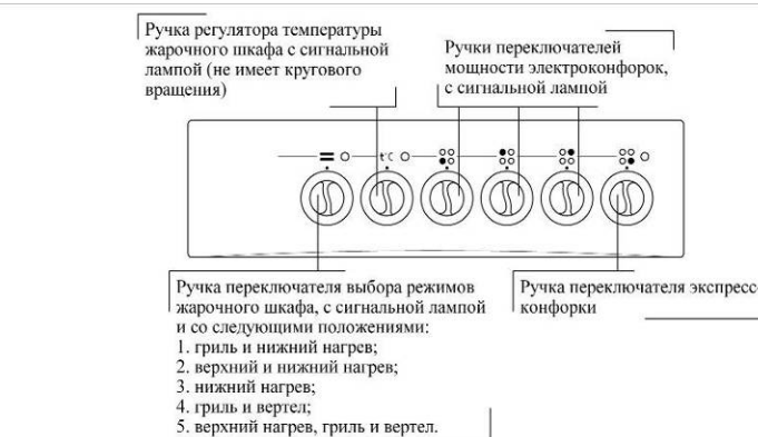
Рис. 12. Передняя панель плиты ЭП4/1э03МС, ЭП4/1э03М2С
