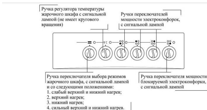
Рис. 11. Передняя панель плиты ЭП411МС, ЭП411М2С
